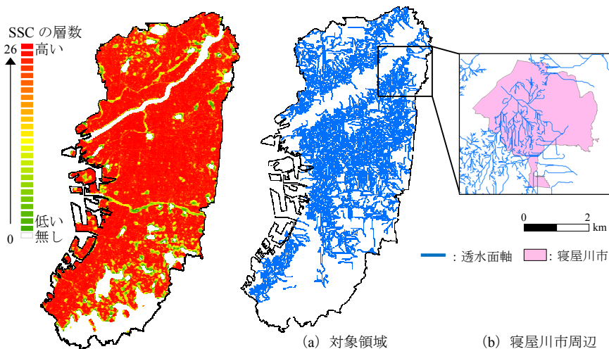
図-2 対象領域での正のSSC
