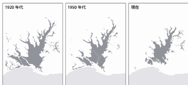
図 3. 釧路湿原の変遷
