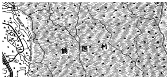
図 2. 地形図上の湿原
